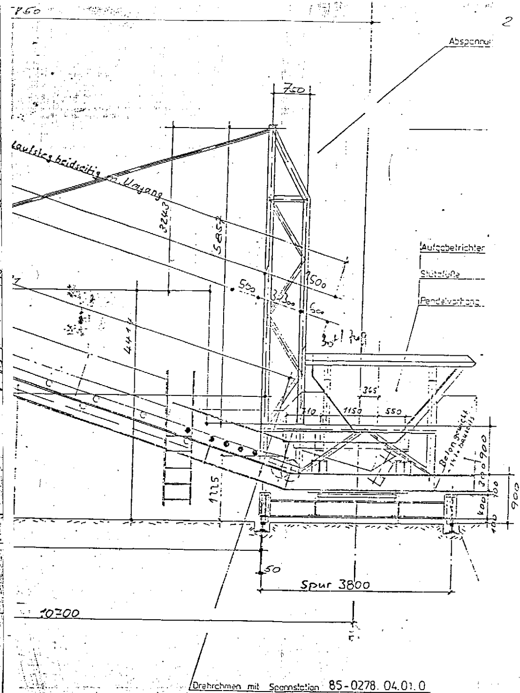
Übersicht zur Statik M 1:100
