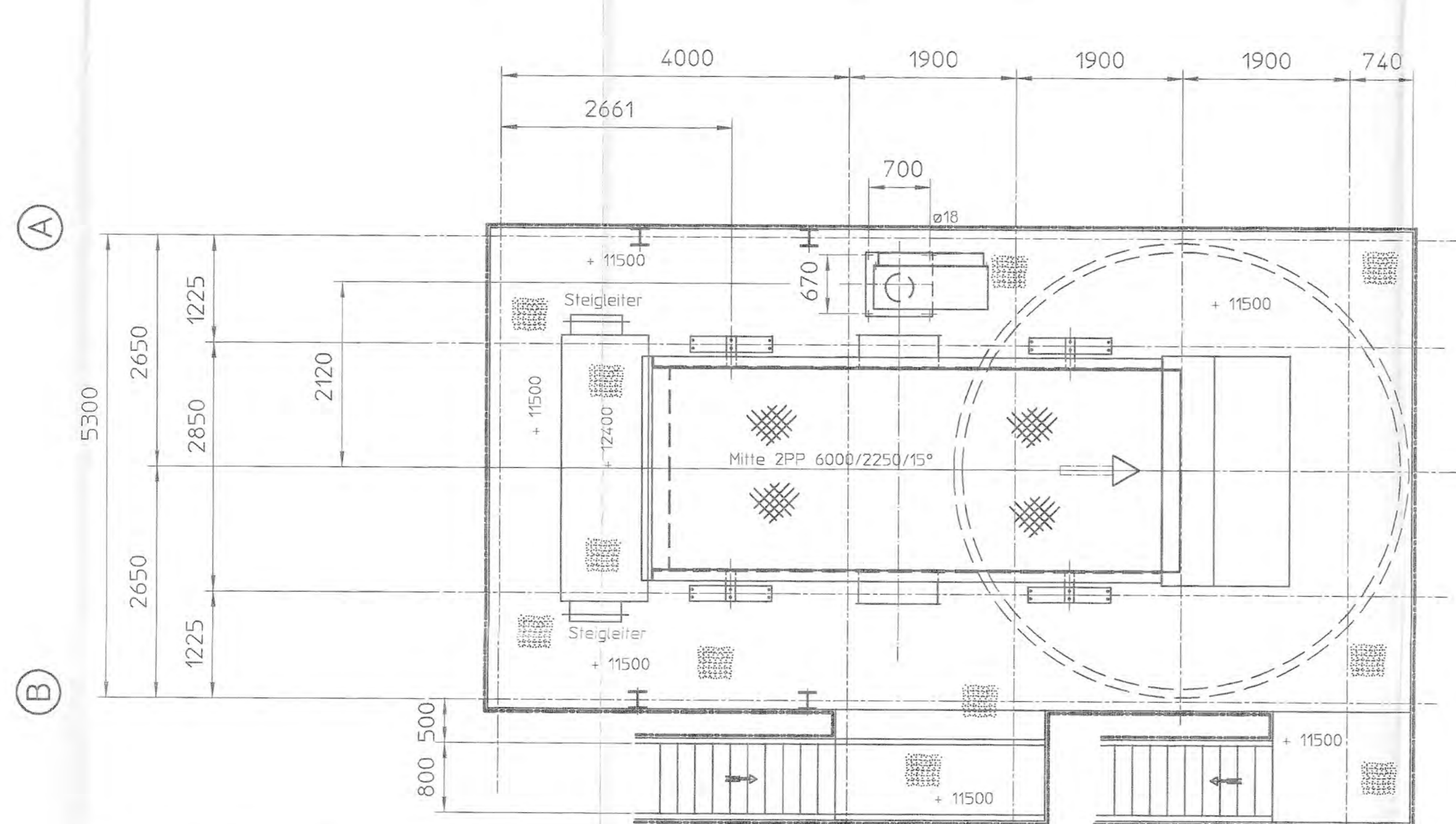
Bühne + 11500
