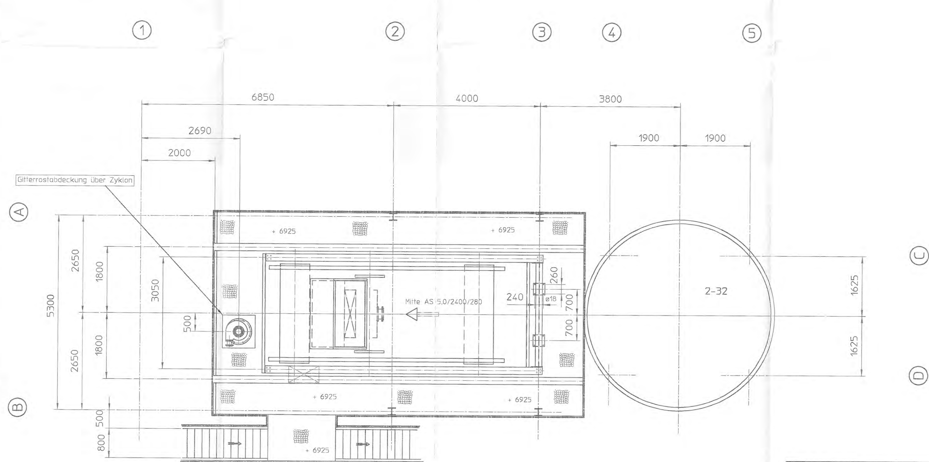
Bühne + 6925
