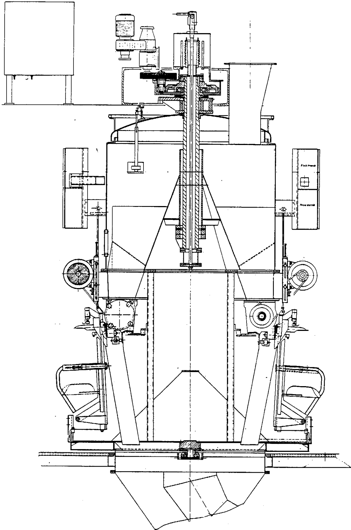
HAYER ROTO PACKER RS (FE)
