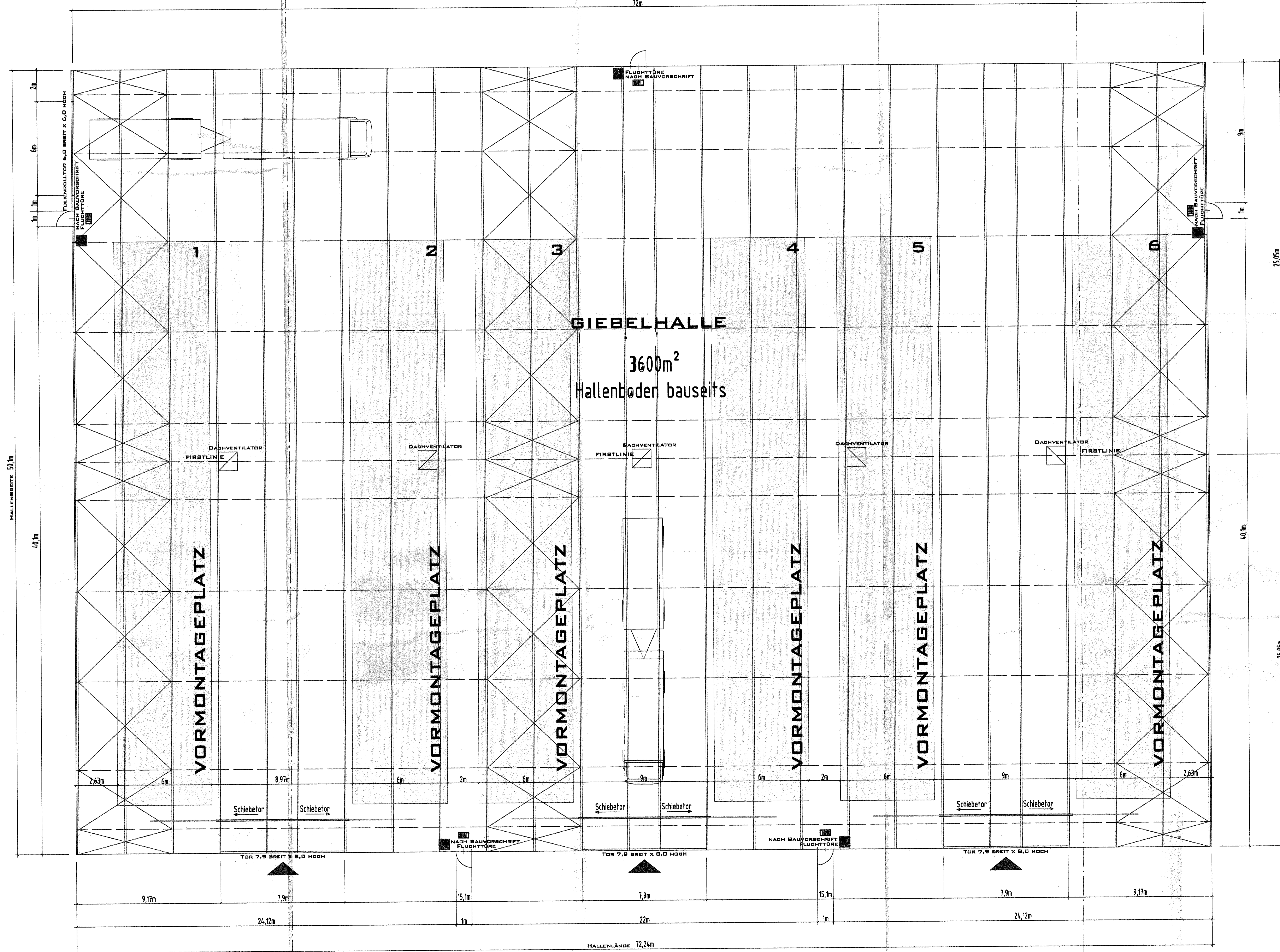
GRUNDRISS
