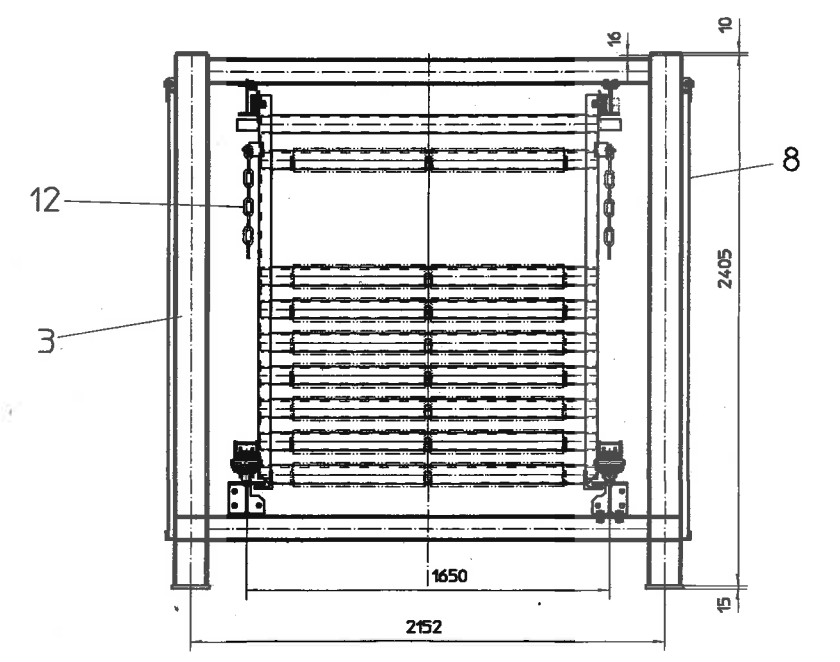
Schnitt A-A M1:20
