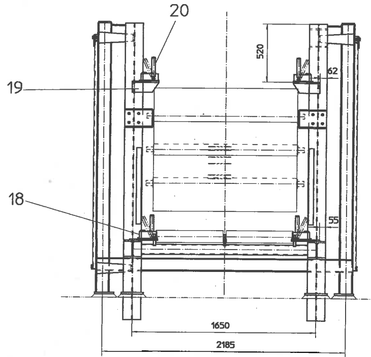
Schnitt B-B M1:20
