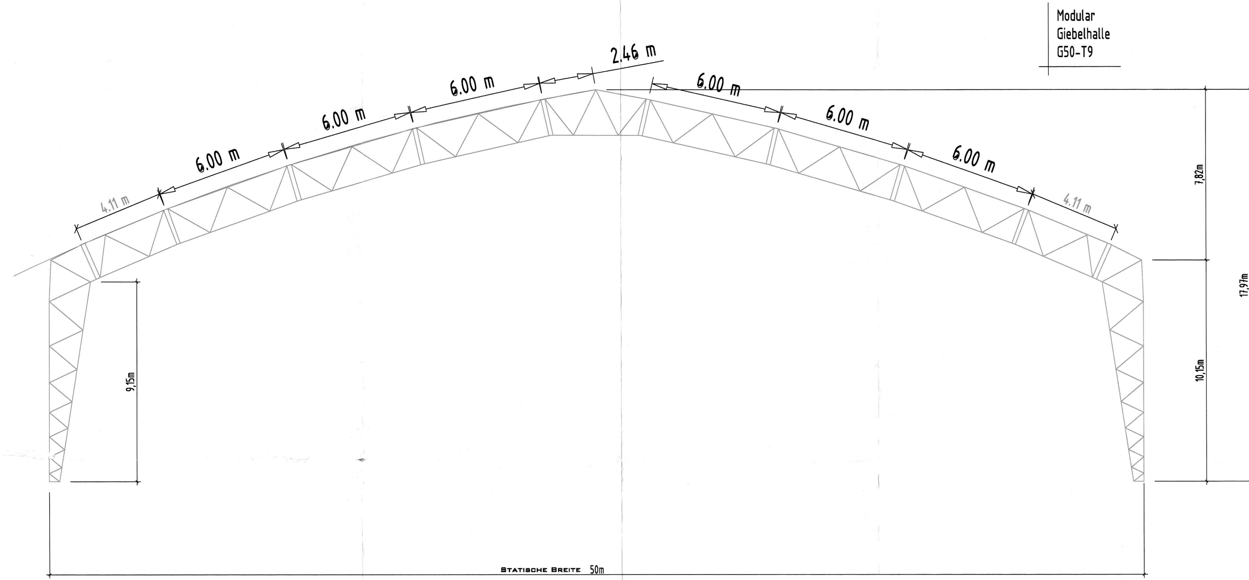
SYSTEMLINIE STATIK
