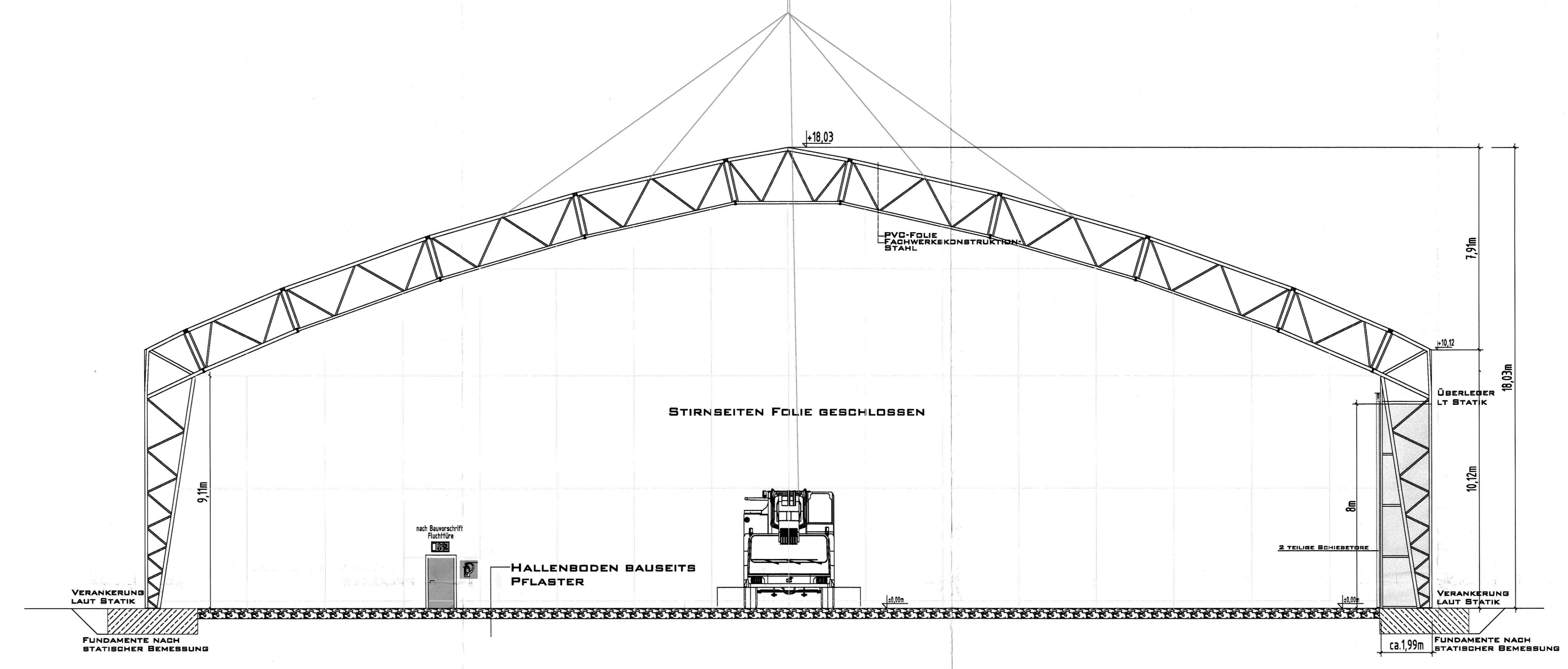
SCHNITT A-A
