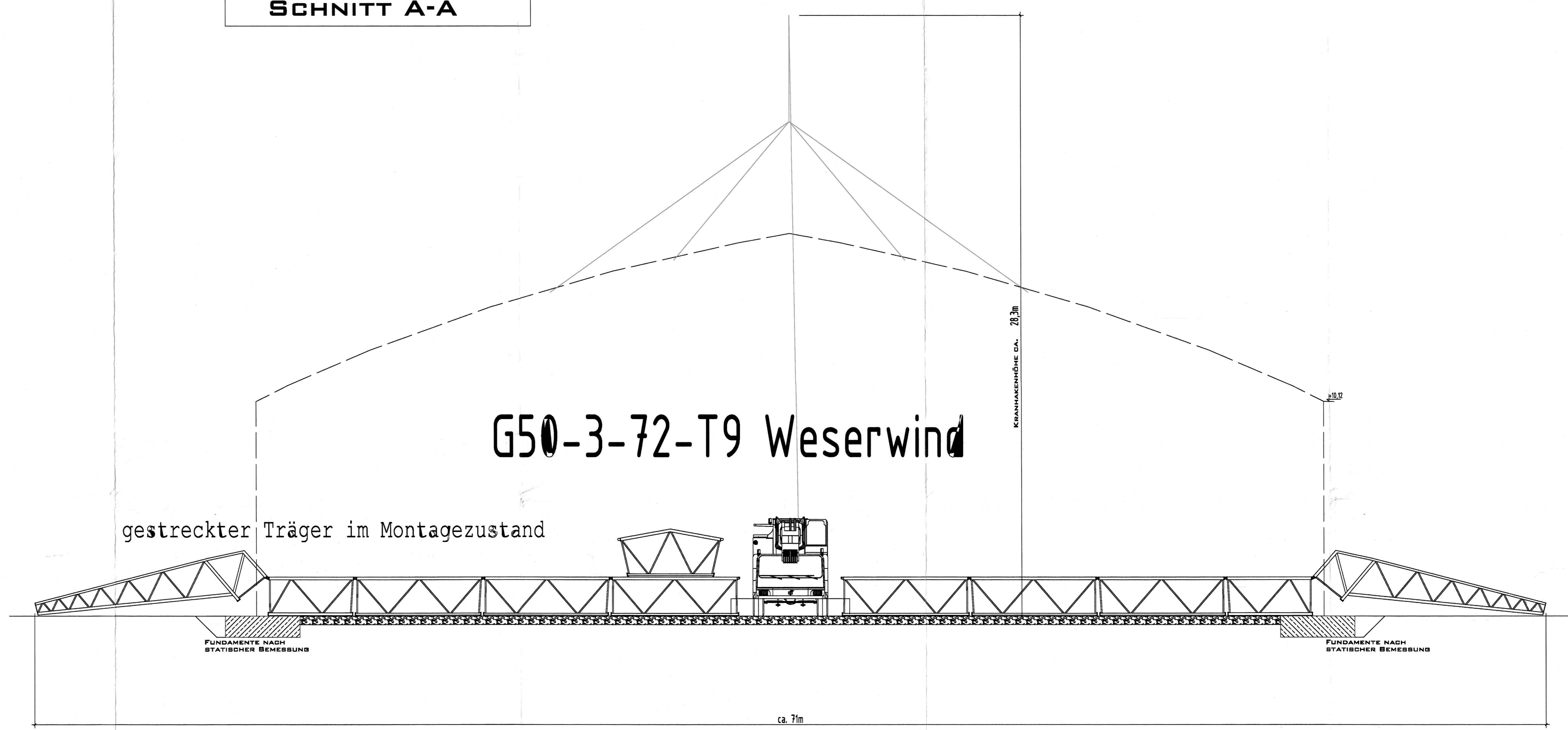
MONTAGEZUSTAND
